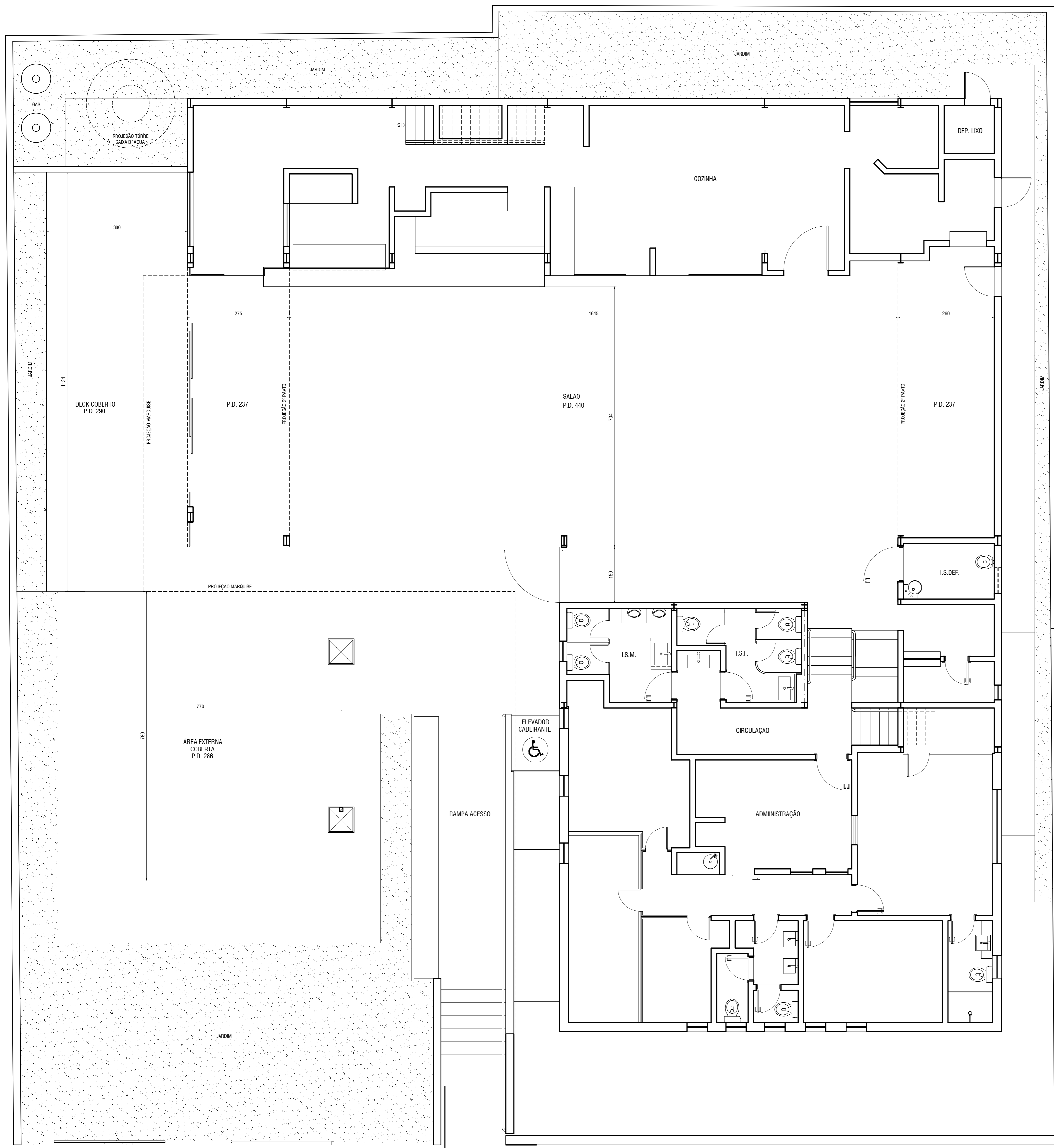
PLANTA PAVTO, TÉRREO ESCALA 1:100
