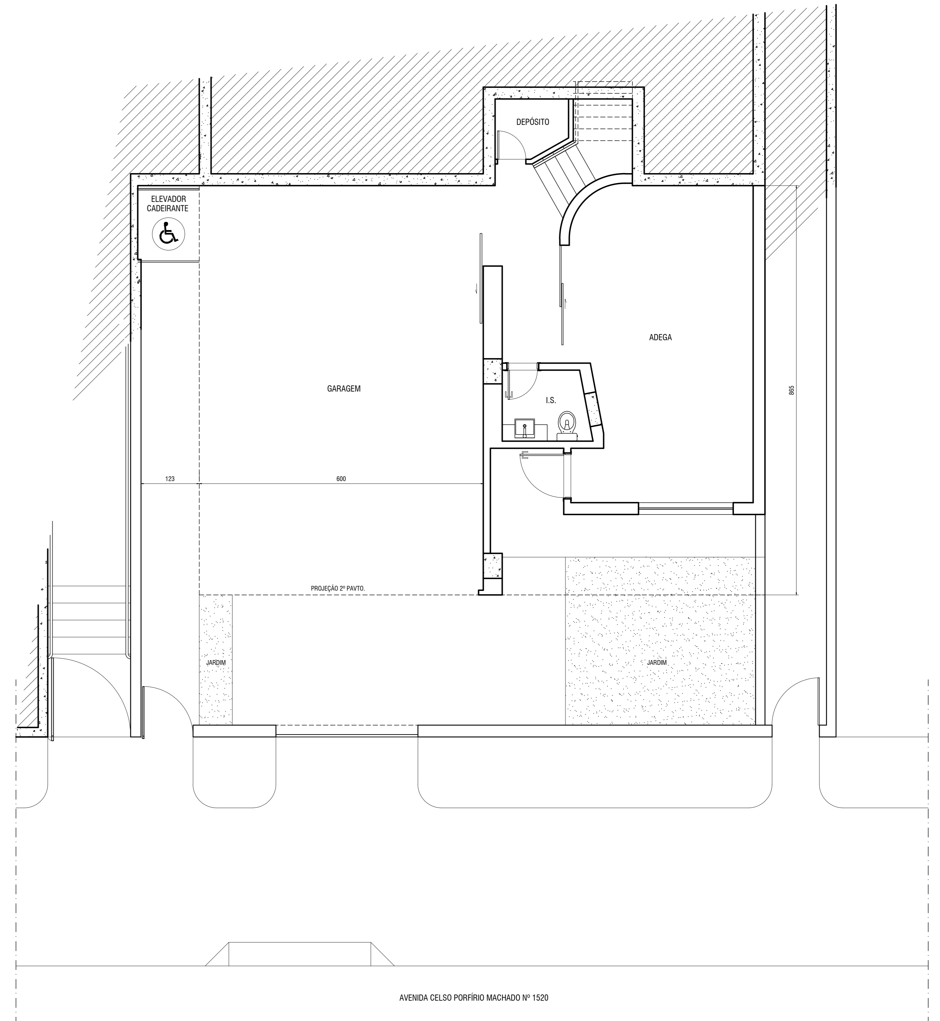
PLANTA PAVTO, INFERIOR ESCALA 1:50
